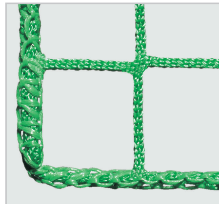
obšití lemu síťe 5 - 7 mm
