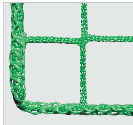
obšití lemu sítě 5 - 7 mm
